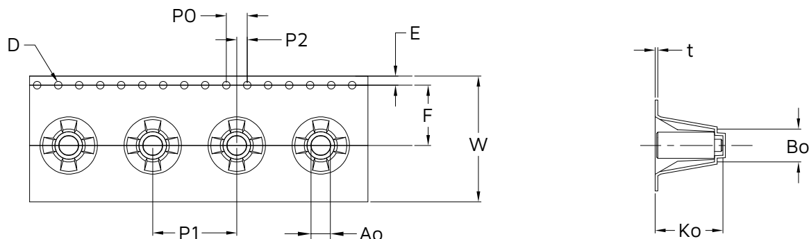
REEL DIMENSIONS
